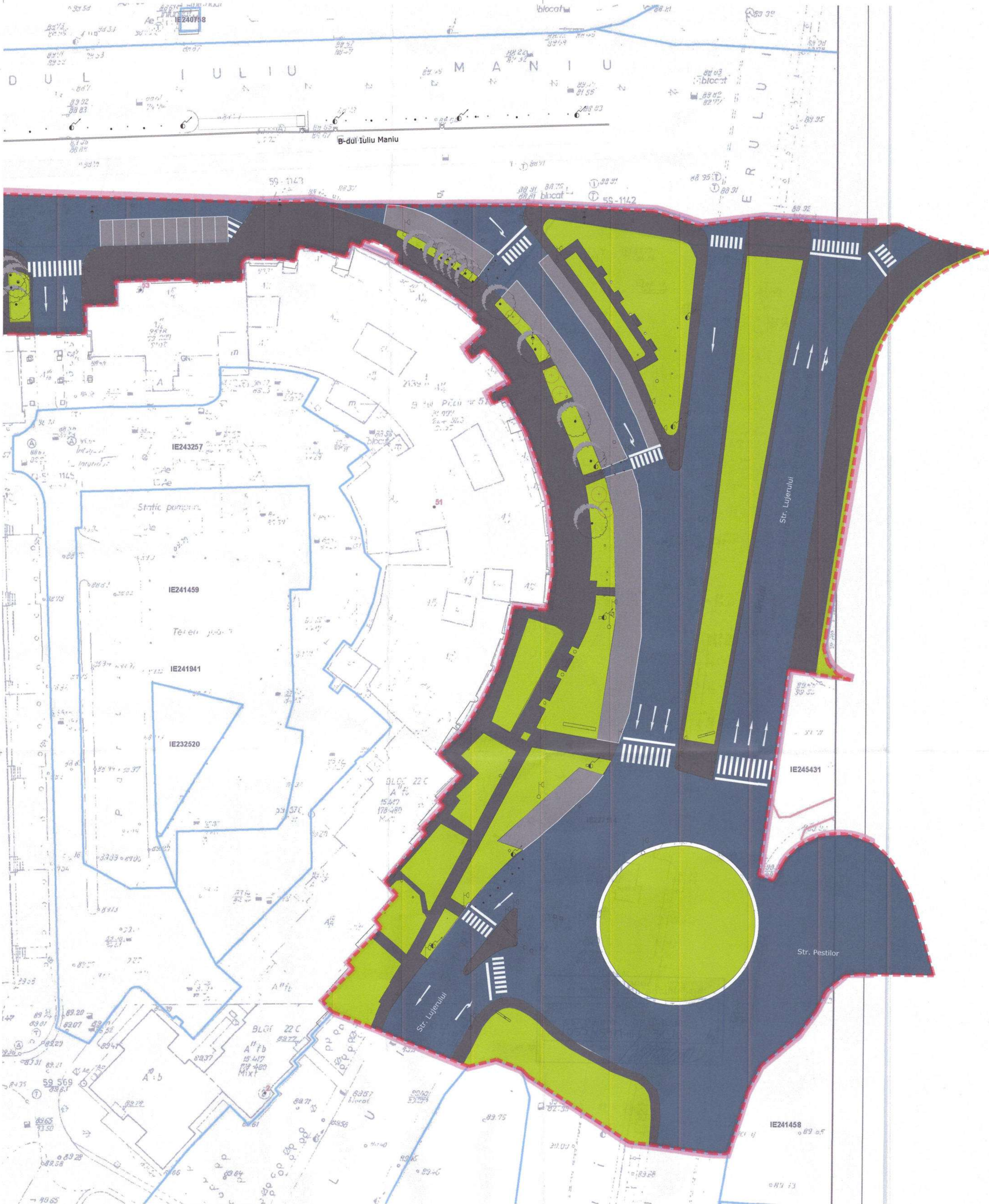
PLAN DE SITUATIE - Tronson Lujerului 1 : 500
