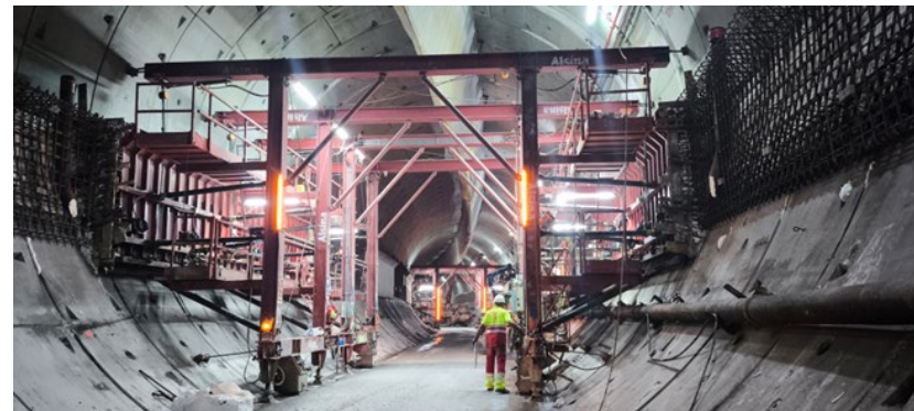
Carros encofrat Tram Lesseps
