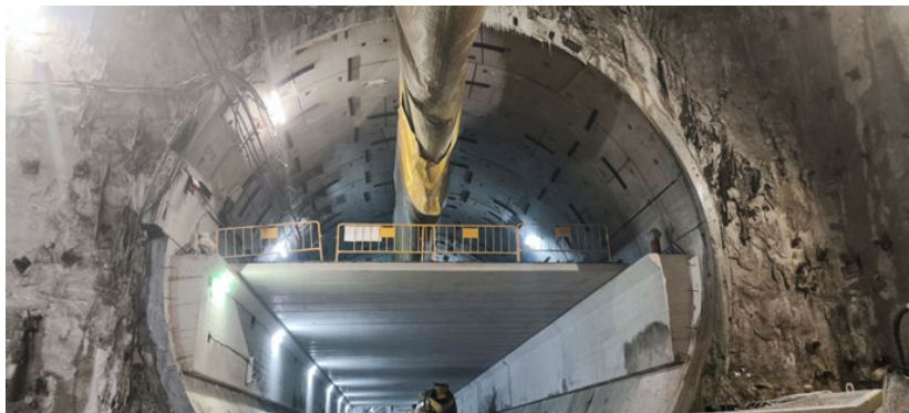
Secció superior túnel a galeria de Guinardó
